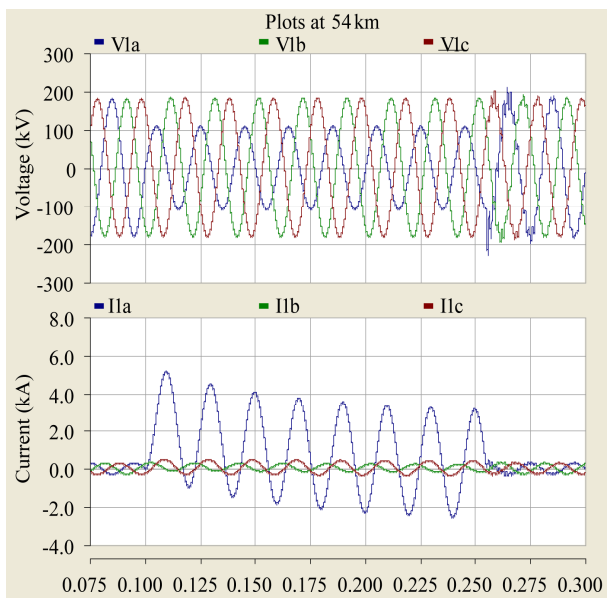
Figure 3. The substation A 54 km A phase voltage, current curve 图 3. 距变电站 A 54 km 处 A 相的电压、电流波形
