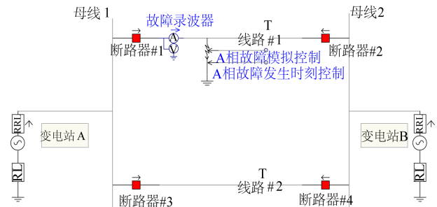
Figure 1. Simulation model 图 1. 仿真模型
