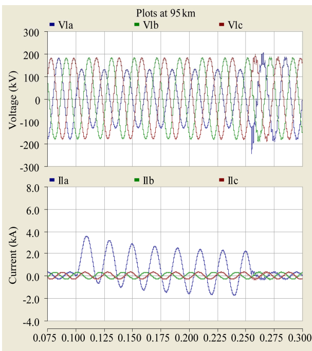
Figure 4. The substation A 95 km A phase voltage, current curve 图 4. 距变电站 A 95 km 处 A 相的电压、电流波形
