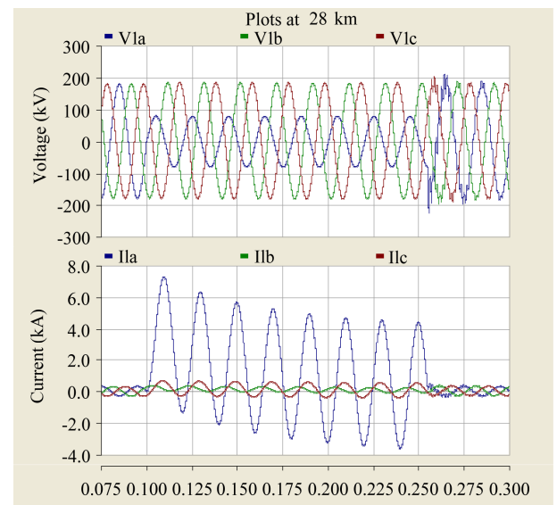
Figure 2. The substation A 28 km A phase voltage, current curve 图 2. 距变电站 A 28 km 处 A 相的电压、电流波形
