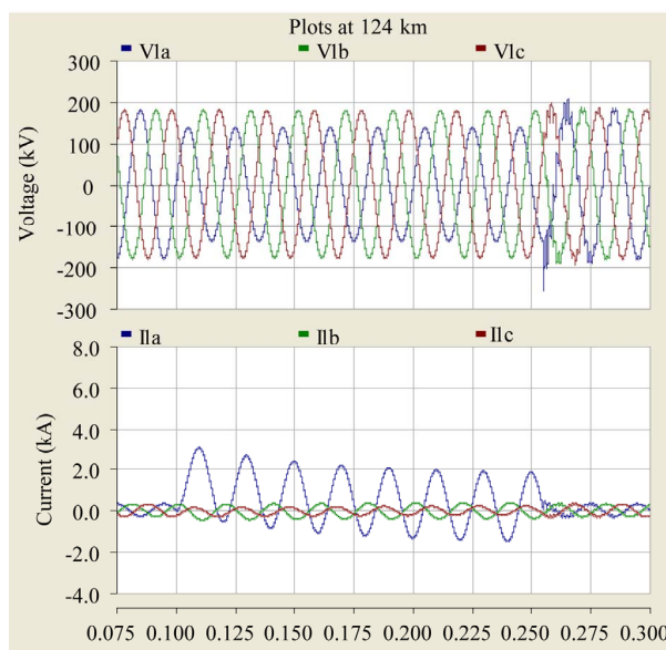
Figure 5. The substation A 124 km A phase voltage, current curve 图 5. 距变电站 A 124 km 处 A 相的电压、电流波形
