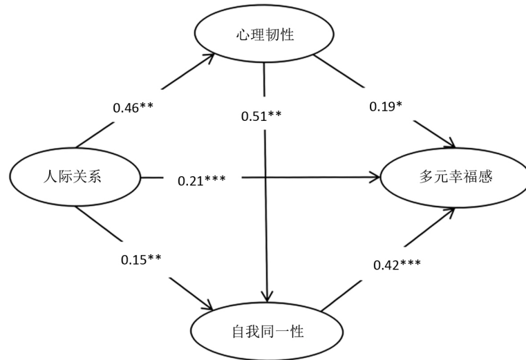
Figure 1. Chained mediation model 图 1. 链式中介模型
