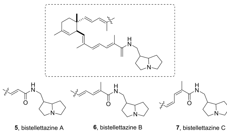
Figure 4. Pyrrolizidine alkaloid bistellettazine A-C 图 4. 吡咯里西啶生物碱 bistellettazine A-C
