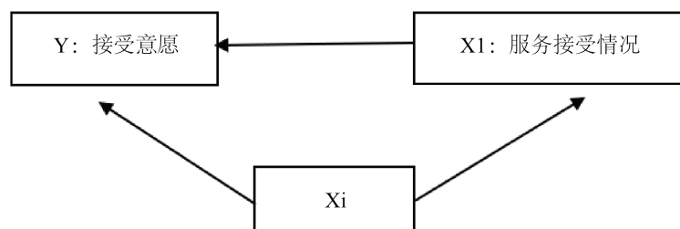
Figure 1. Propensity score matching schematic diagram 图 1. 倾向得分匹配原理说明图
